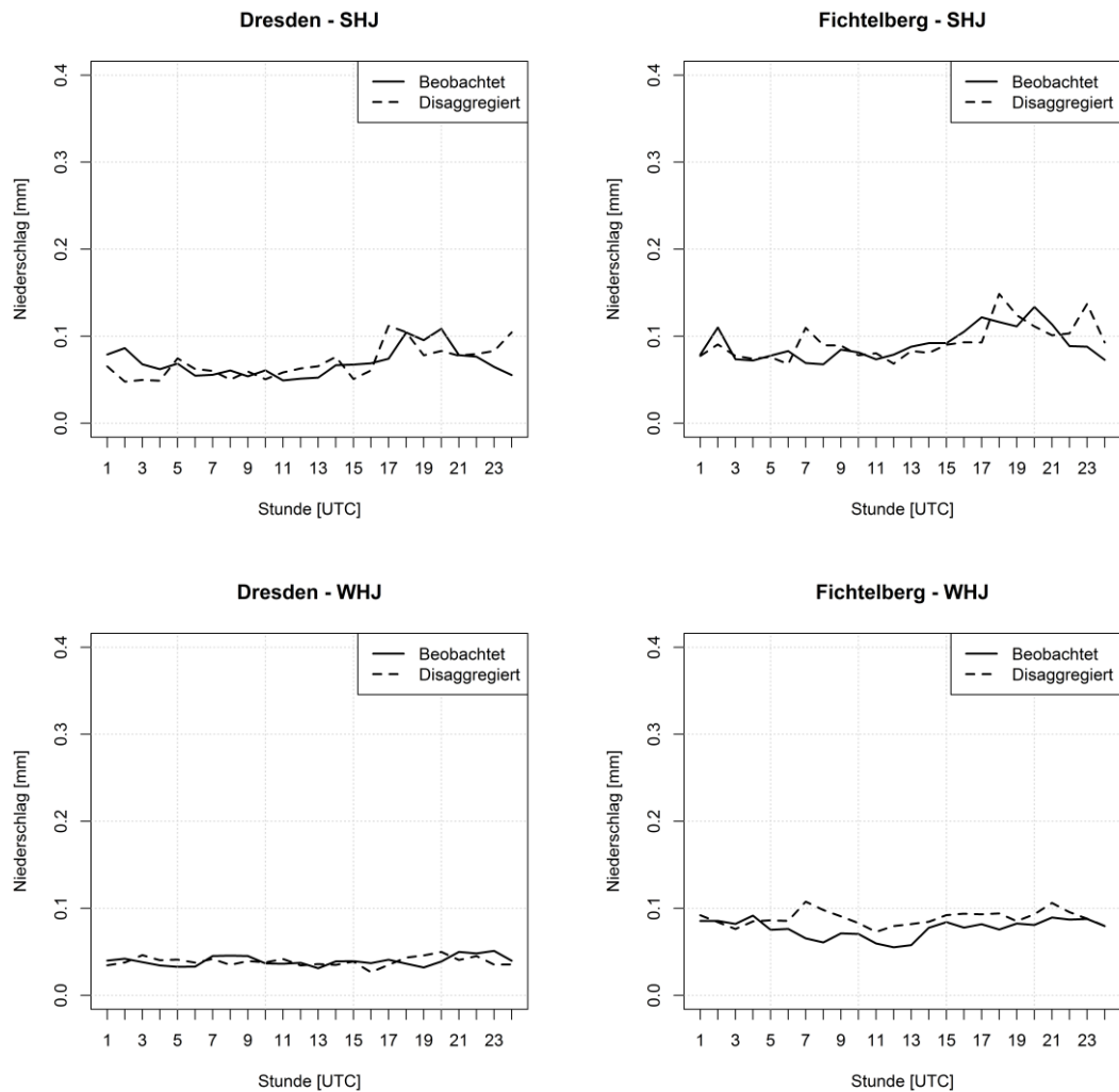
Abbildung 3: Beobachtete und disaggregierte Tagesgänge des Niederschlags für Dresden-Klotzsche (links) und Fichtelberg (rechts), Sommerhalbjahr SHJ und Winterhalbjahr WHJ
