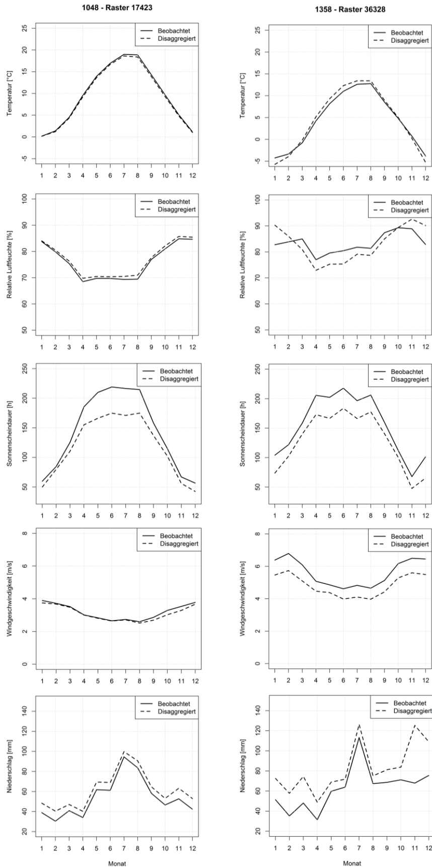
Abbildung 7: Jahresgang der beobachteten stündlichen Werte und der nächstgelegenen disaggregierten Rasterzelle des Referenzdatensatzes an den Stationen Dresden-Klotzsche (links) und Fichtelberg (rechts)
