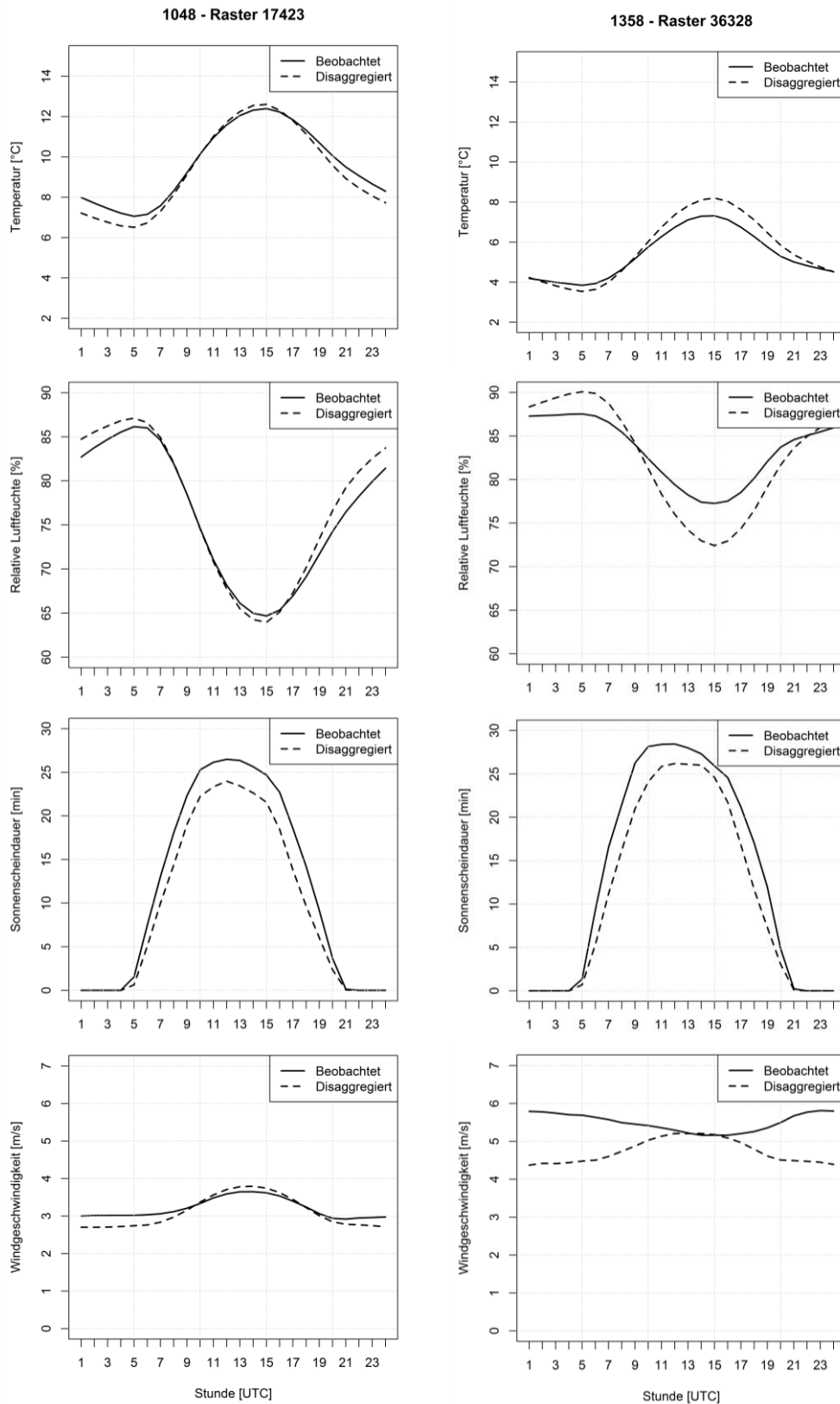
Abbildung 5: Tagesgang der beobachteten stündlichen Werte und der nächstgelegenen disaggregierten Rasterzelle des Referenzdatensatzes an den Stationen Dresden (links) und Fichtelberg (rechts), Jahresmittel
