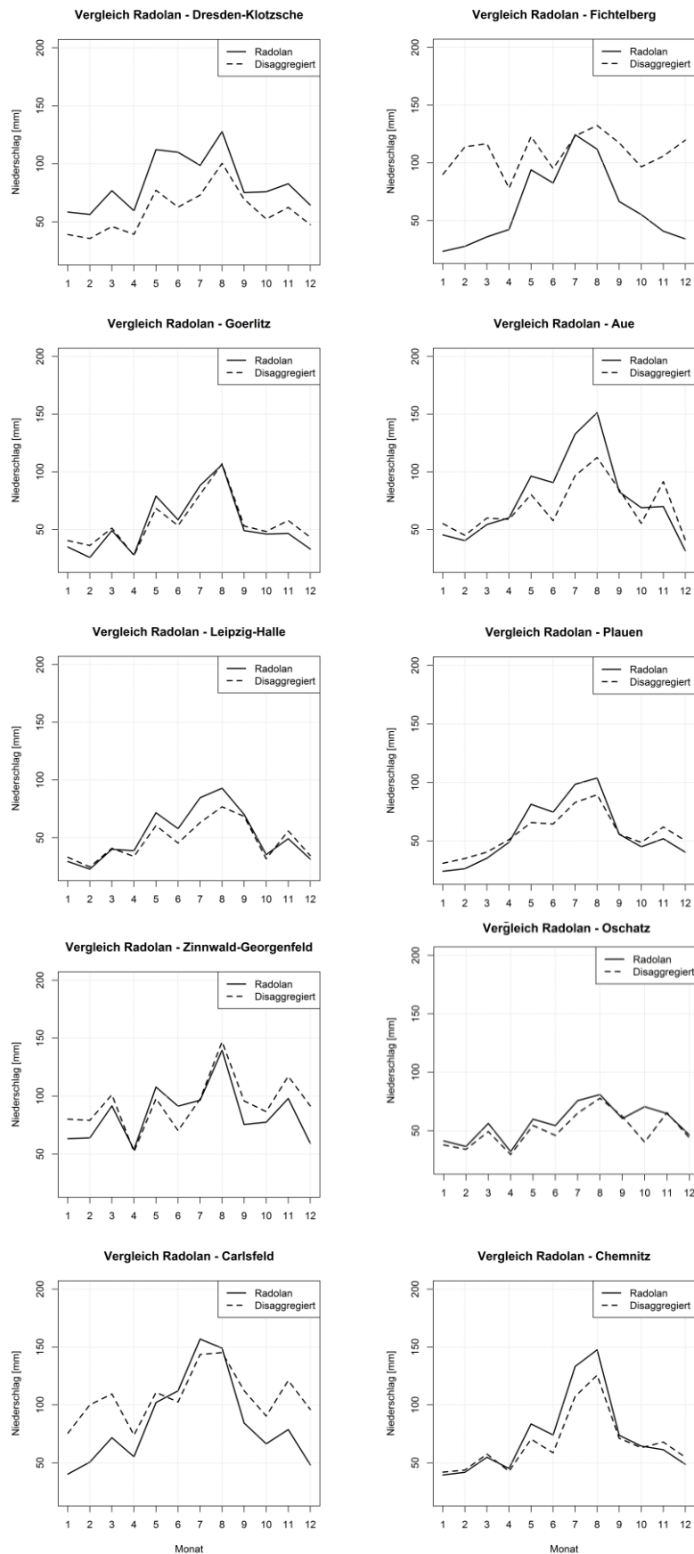
Abbildung 9: Vergleich der Jahresgänge, gebildet aus disaggregierten Niederschlägen von zehn Klimastationen und beobachteten Radarwerten
